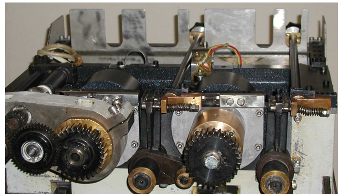
Komplettüberholung einer Klebebinder - Rückenbeleimungsstation
